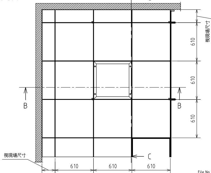
平面組裝示意圖
