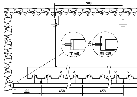
A-A 詳剖圖
