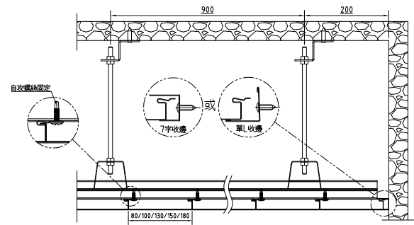
B-B 詳剖圖
